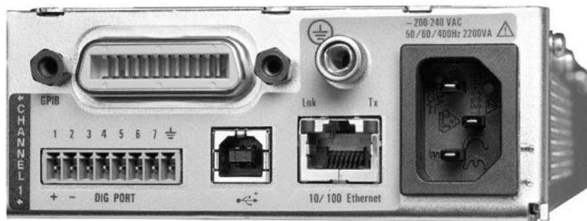
Рисунок 1 - Стандартные средства подключения: интерфейсы GPIB, 10/100 Base-T Ethernet и USB 2.0
