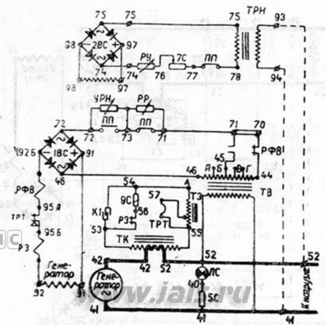
Принципиальная схема агрегата типа АЛА-3,5-М
